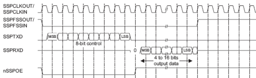
Рисунок 109 – Формат синхронного обмена протокола Microwire (одиночный обмен)
