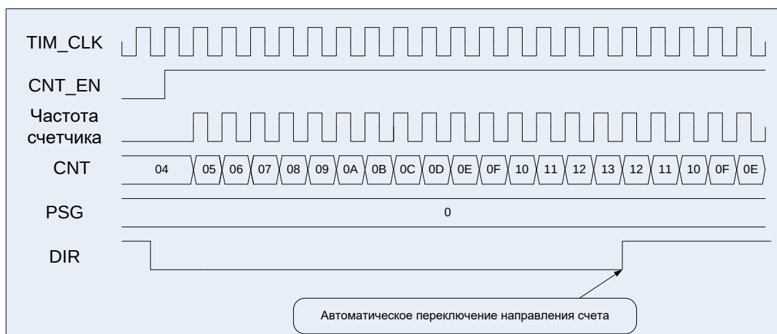
Рисунок 66 – Диаграммы работы таймера, счет двунаправленный, сначала прямой
