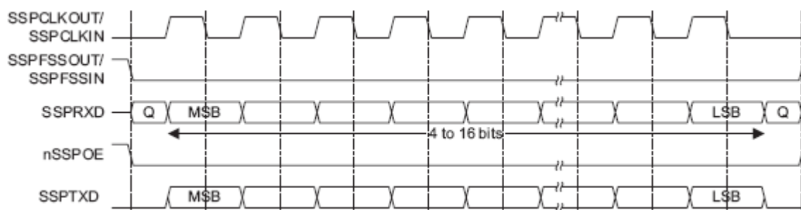
Рисунок 105 – Формат синхронного обмена протокола SPI, SPO=0, SPH=1
