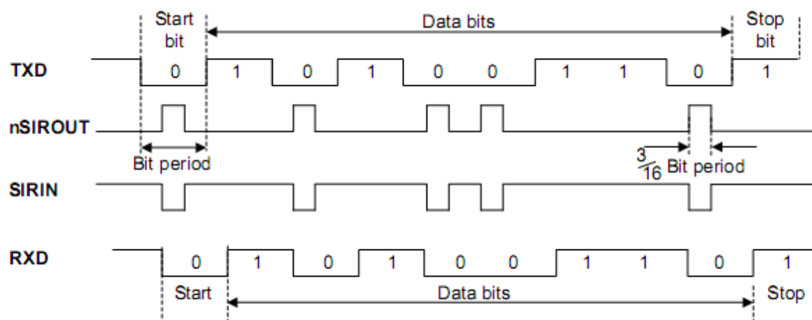
Рисунок 120 – Модуляция данных IrDA
