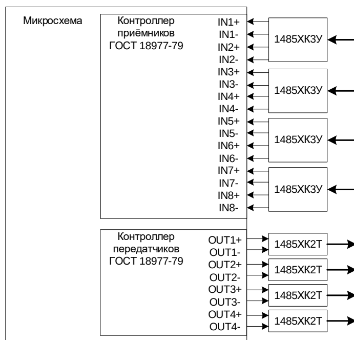
Рисунок 96 – Структура блока контроллера интерфейса по ГОСТ 18977-79
