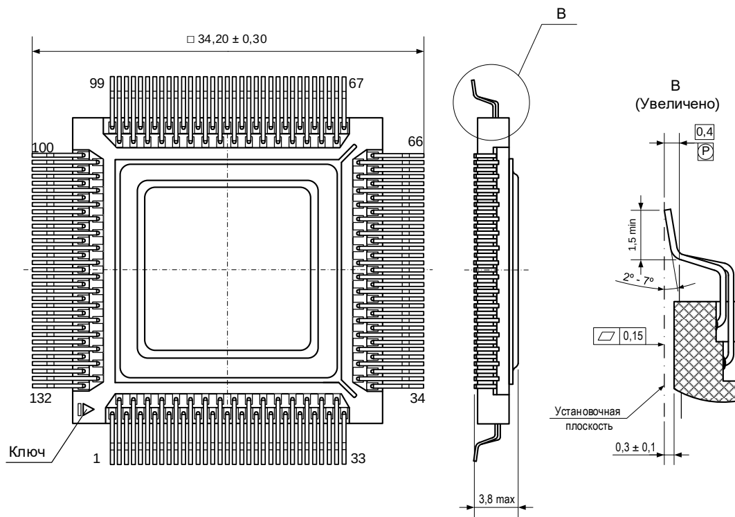
Рисунок 153 – Габаритный чертеж микросхемы в корпусе с формованными выводами
