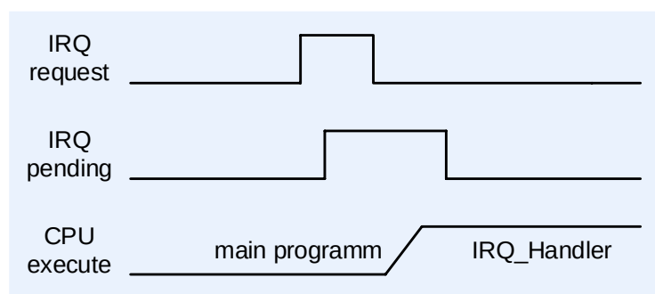
Рисунок 140 – Выставление отложенного запроса на прерывание и последующая его обработка
