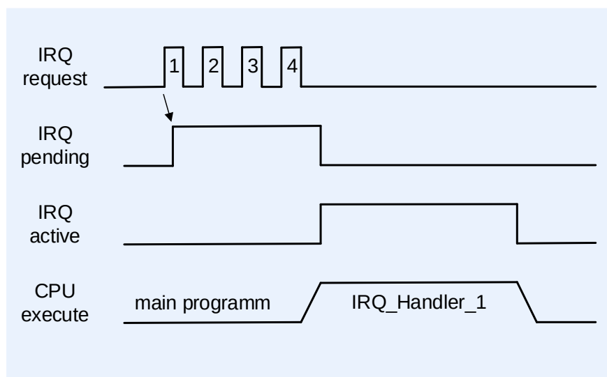
Рисунок 144 – Многократная установка снятие запроса IRQ request
