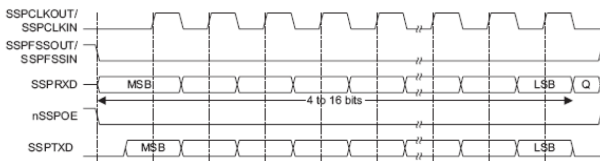
Рисунок 103 – Формат синхронного обмена протокола SPI, SPO=0, SPH=0 (одиночный обмен)
