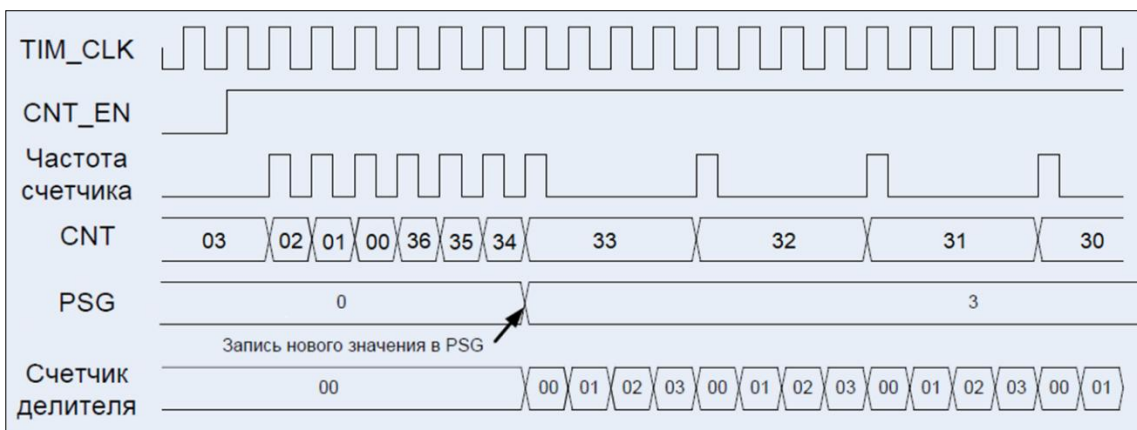
Рисунок 72 – Диаграмма работы счетчика: счет обратный (CNT_MODE[1:0] = 00, EVENT_SEL[3:0] = 0000, DIR = 1)
