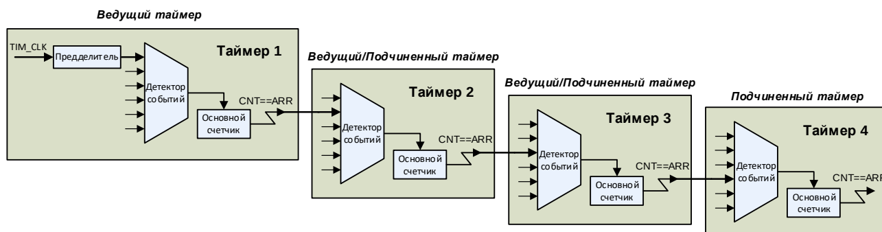
Рисунок 73 – Пример каскадного соединения таймеров
