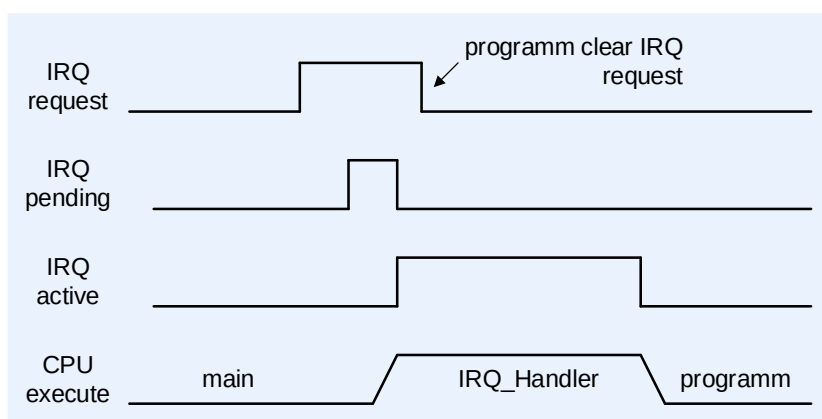
Рисунок 142 – Сброс признака отложенного прерывания, до обработки ядром
