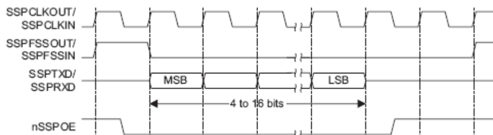
Рисунок 101 – Формат синхронного обмена протокола SSI (единичный обмен)
