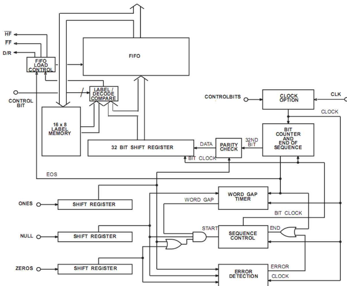
Рисунок 98 – Структурная схема канала приема
