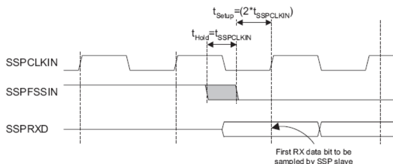
Рисунок 111 – Формат Microwire, требования к времени установки и удержания сигнала SSPFSSIN
