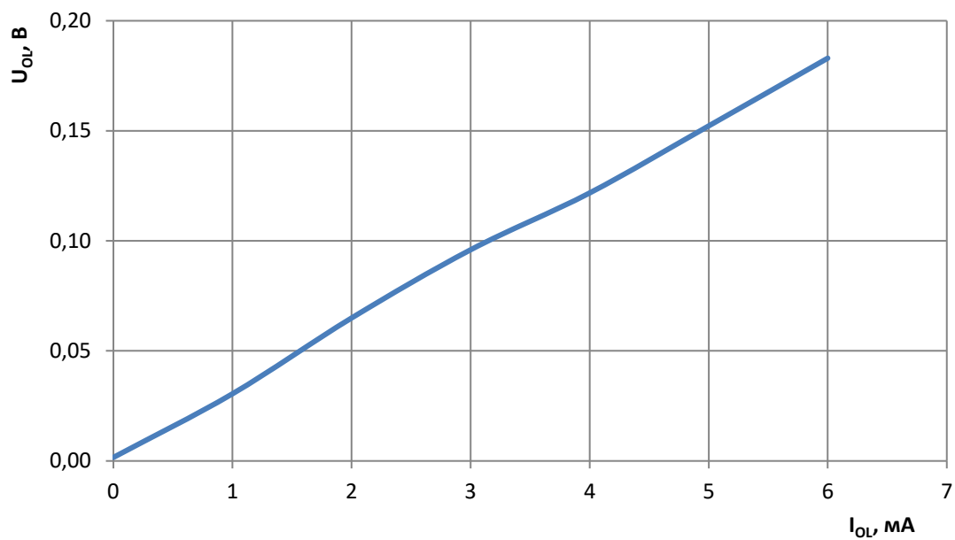
Рисунок 151 – Зависимость выходного напряжения низкого уровня от выходного тока низкого уровня при напряжении питания 3,0 В
