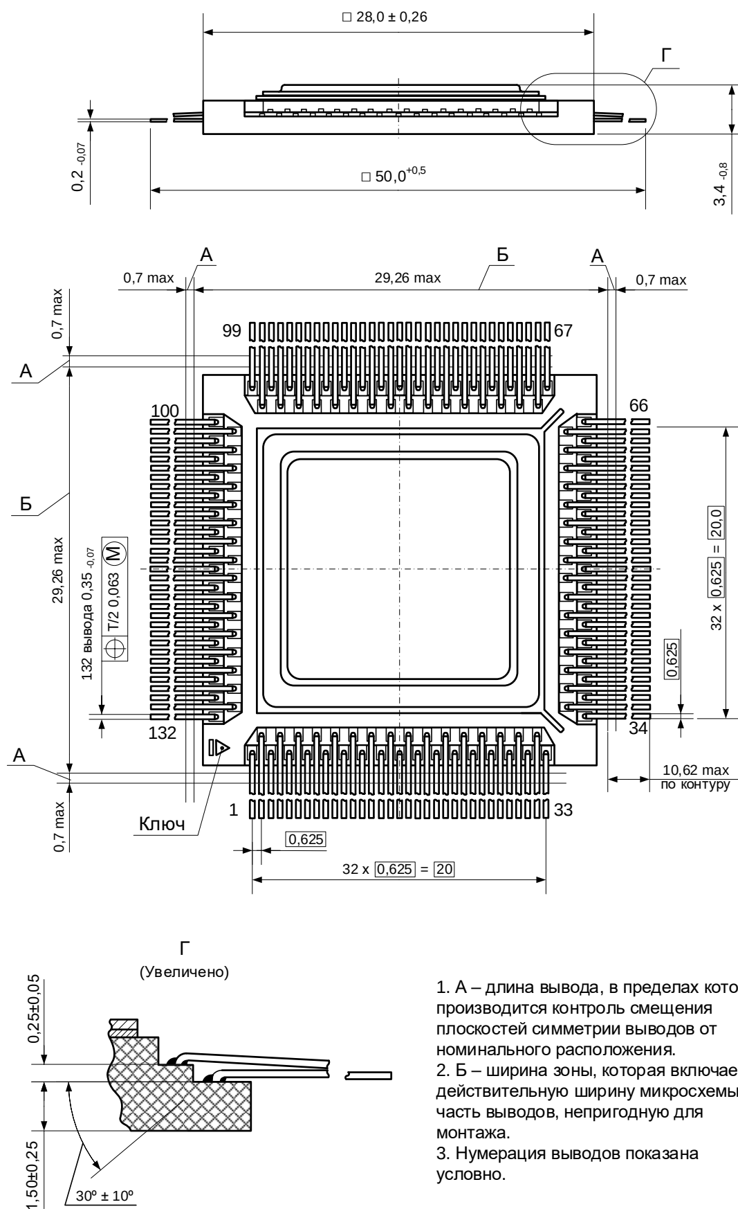
Рисунок 152 – Габаритный чертеж микросхемы в корпусе 4229.132-3
