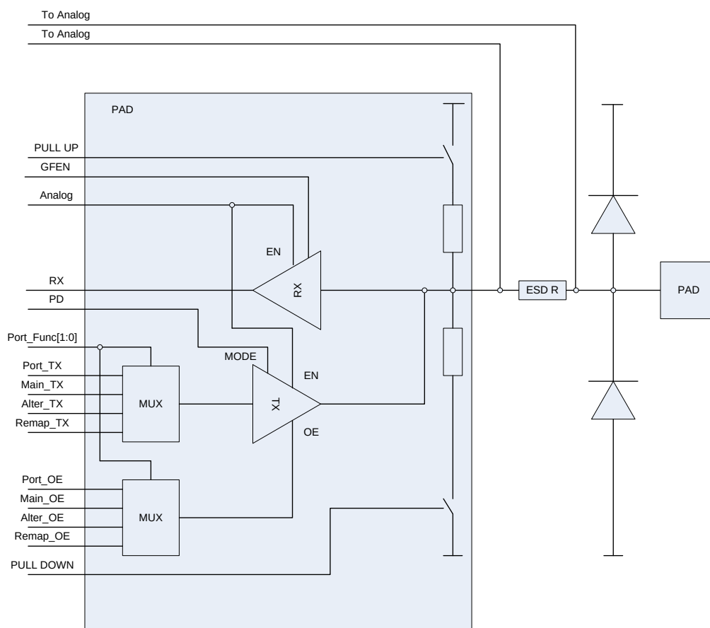
Рисунок 26 – Порты ввода/вывода
