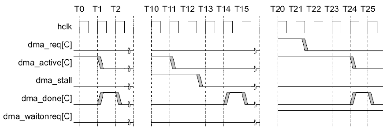
Рисунок 126 – Диаграммы функционирования dma_done
