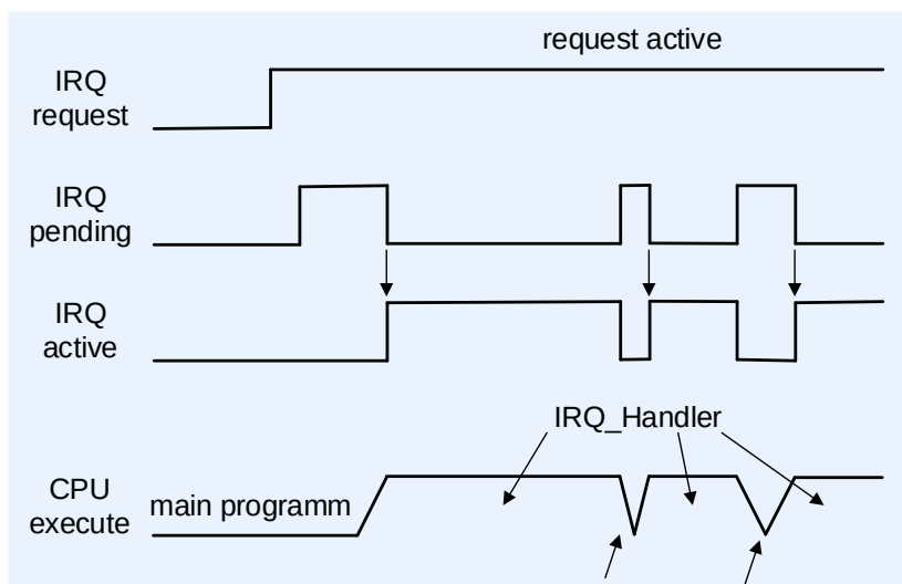
Рисунок 143 – Повторная обработка прерываний при удержании запроса от источника
