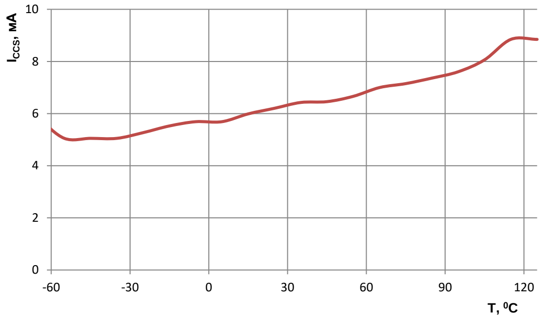
Рисунок 149 – Зависимость статического тока потребления в режиме покоя (регулятор напряжения выключен) от температуры при напряжении U_{CC}=3.6V
