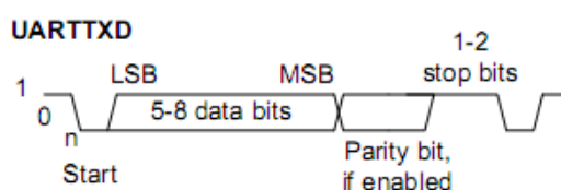
Рисунок 119 – Кадр передачи данных
