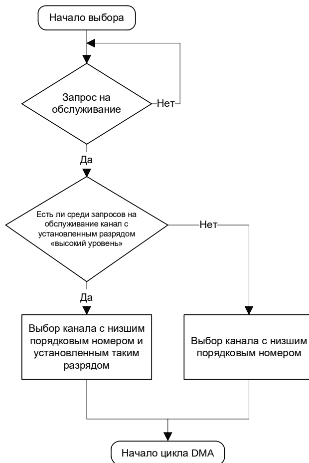
Рисунок 129 – Алгоритм выбора следующего канала для обслуживания
