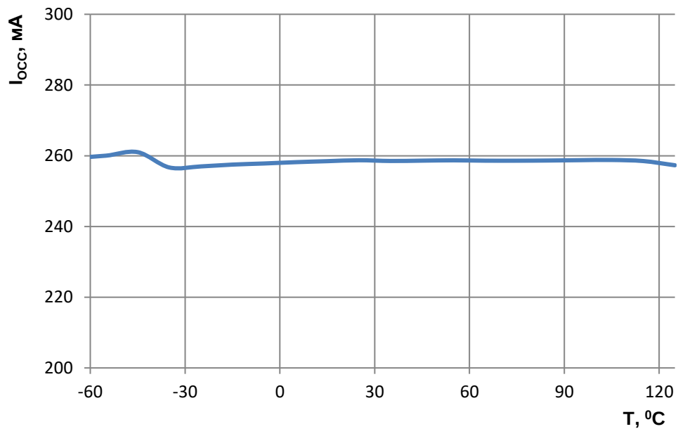
Рисунок 147 – Зависимость динамического тока потребления от температуры при: f_C = 144 МГц
