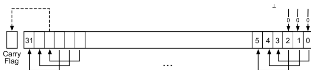
Рисунок 20 – Инструкция LSL \# 3
