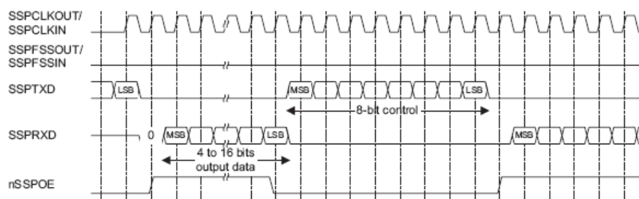
Рисунок 110 – Формат синхронного обмена протокола Microwire (непрерывный обмен)
