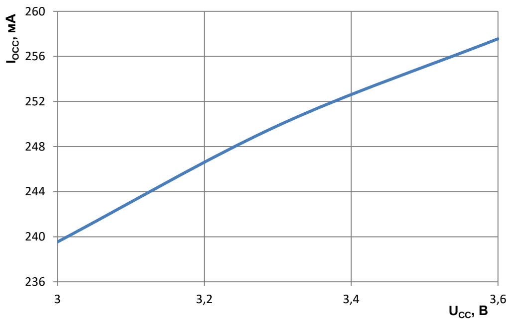
Рисунок 148 – Зависимость динамического тока потребления от напряжения питания
