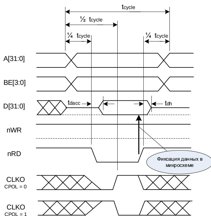
Рисунок 29 – Диаграмма чтения
