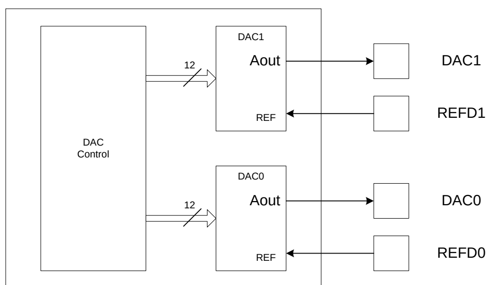
Рисунок 95 – Структурная схема контроллера ЦАП
