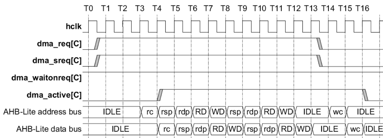
Рисунок 127 – Диаграмма работы контроллера DMA при использовании dma_waitonreq
