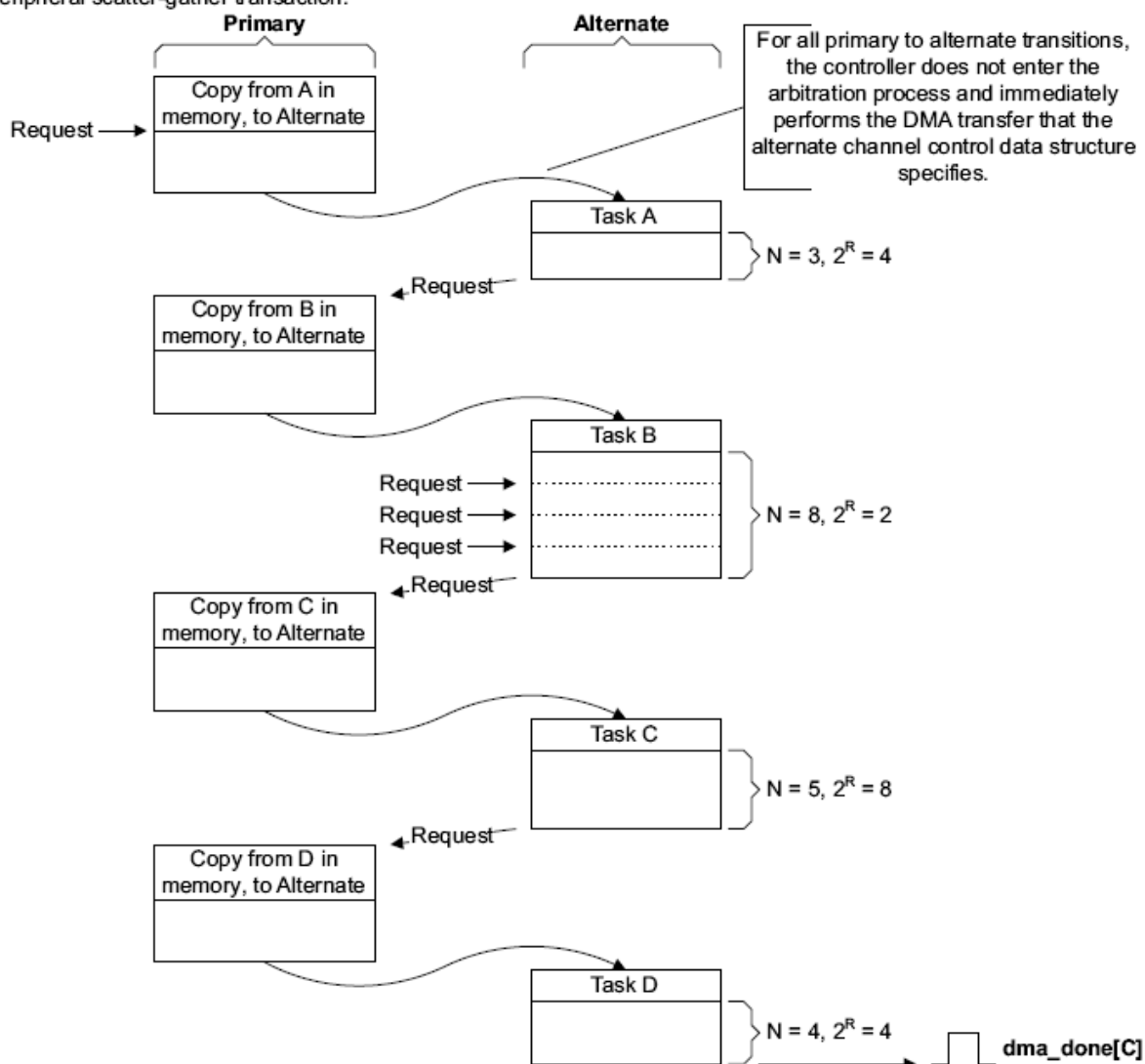
Рисунок 132 – Пример работы DMA в режиме с «Исполнением с изменением конфигурации»
