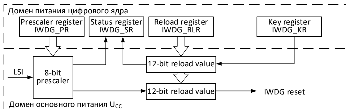
Рисунок 146 – Блок-схема независимого сторожевого таймера
