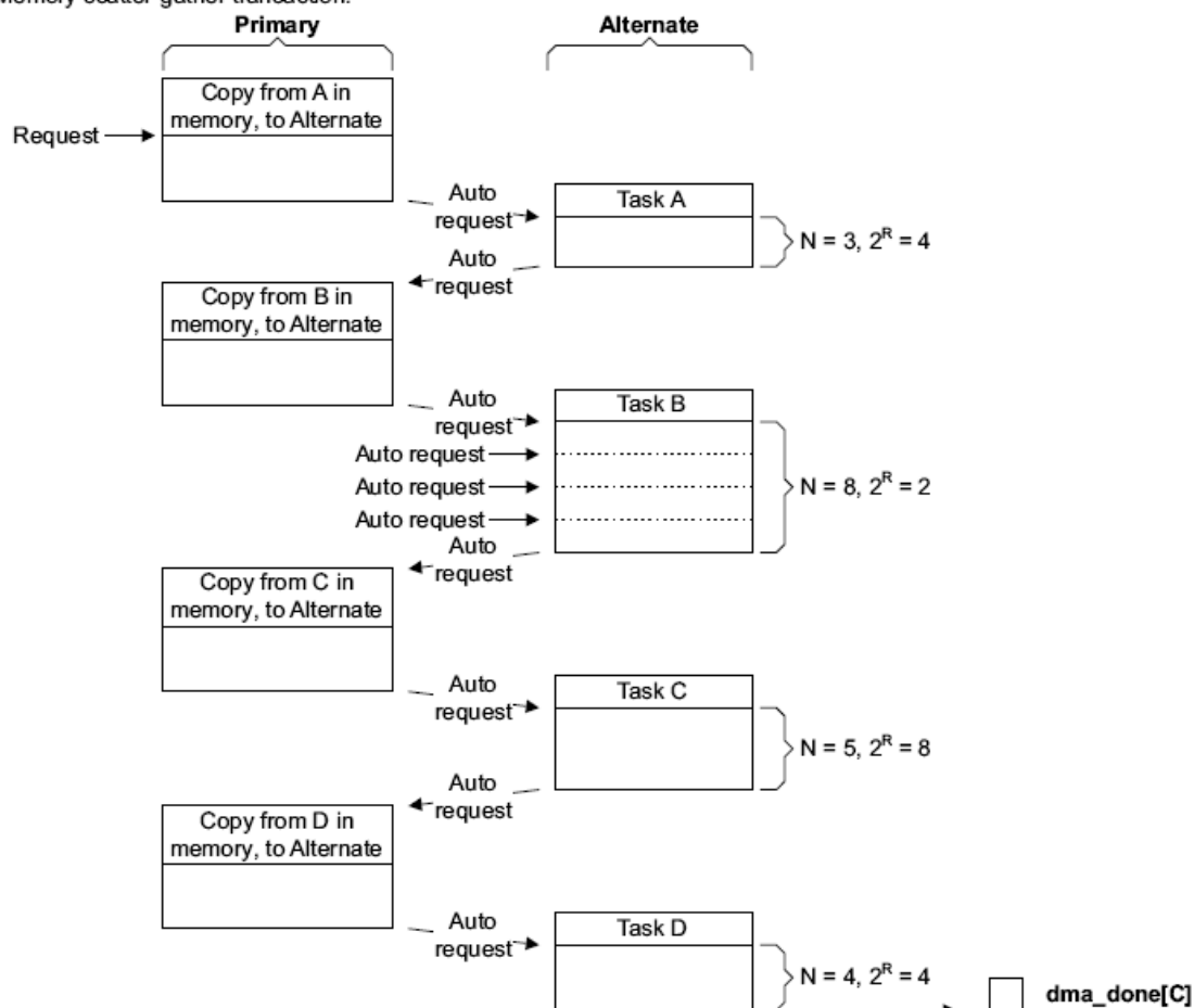
Рисунок 131 – Пример работы DMA в режиме с «Исполнением с изменением конфигурации»
