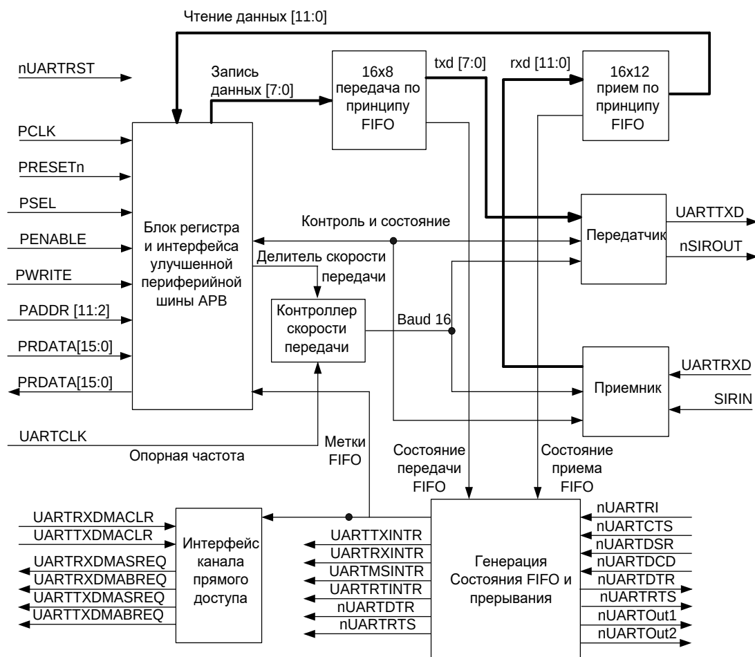
Рисунок 116 – Блок-схема универсального асинхронного приемопередатчика (UART)
