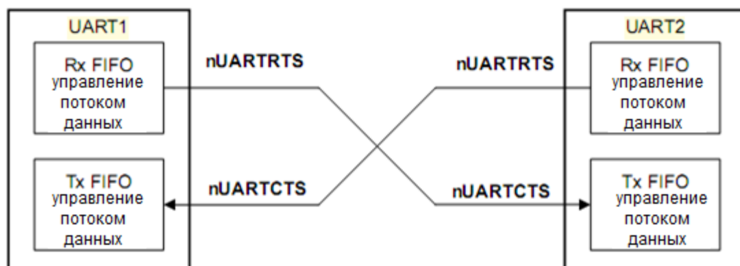
Рисунок 121 – Взаимодействие двух устройств последовательной связи с аппаратным управлением потоком данных
