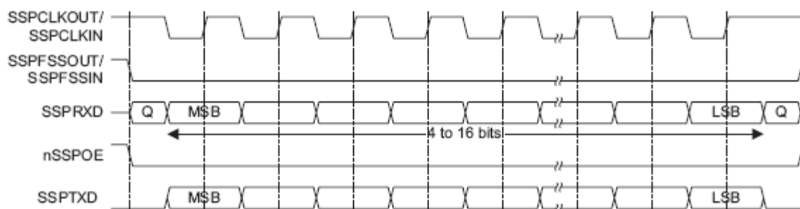
Рисунок 108 – Формат синхронного обмена протокола SPI, SPO=1, SPH=1
