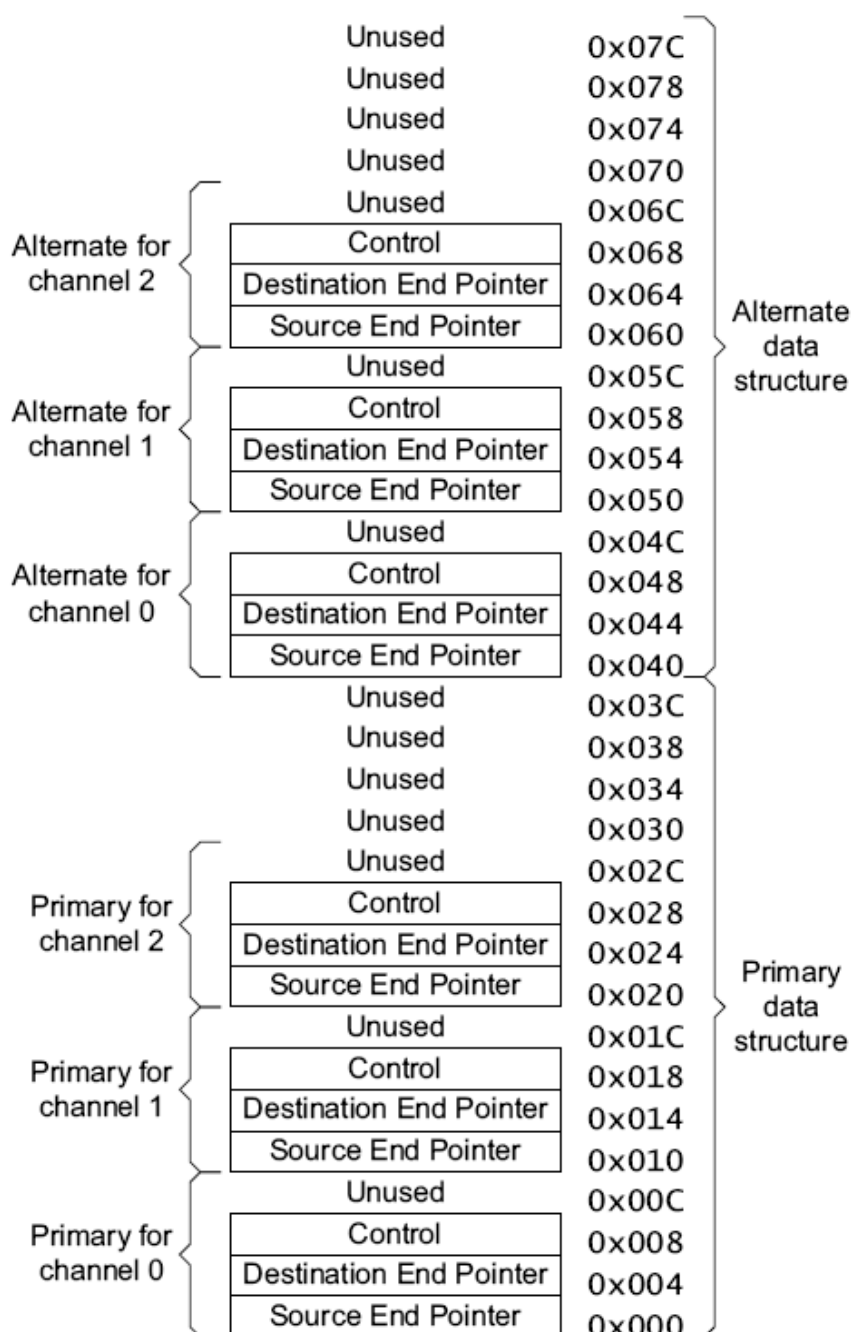
Рисунок 134 – Карта памяти для трех каналов DMA, включая альтернативную структуру управляющих данных (где Destination end pointer – указатель конца данных приемника; Source end pointer – указатель конца данных источника; Control – управление)
