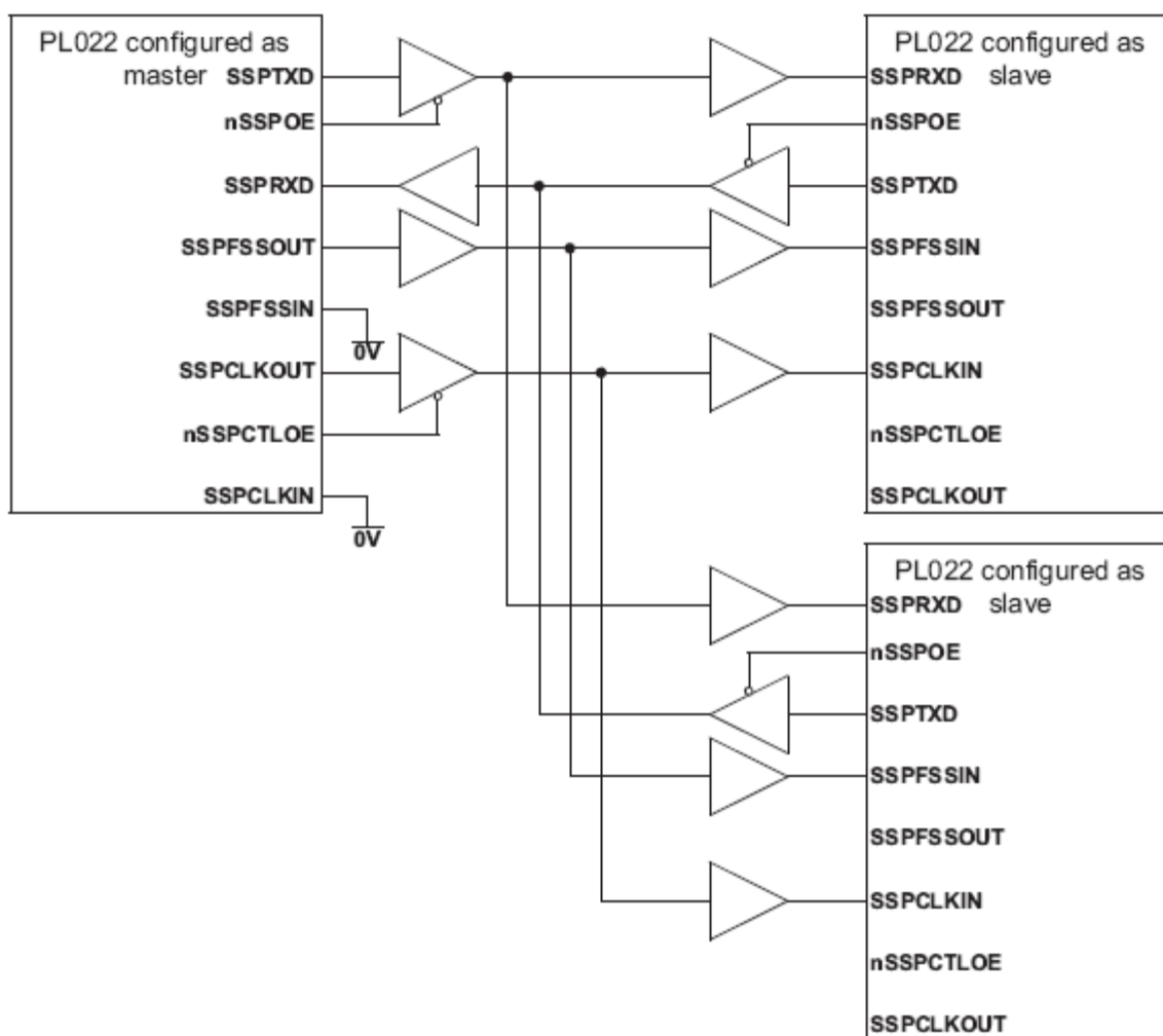
Рисунок 112 – Ведущее устройство SSP подключено к двум ведомым
