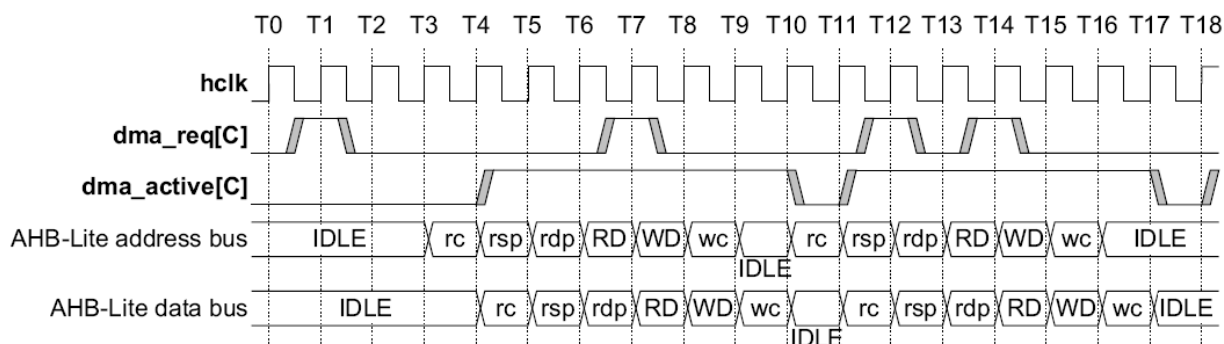
Рисунок 124 – Диаграмма работы при получении импульсного запроса от периферийного блока
