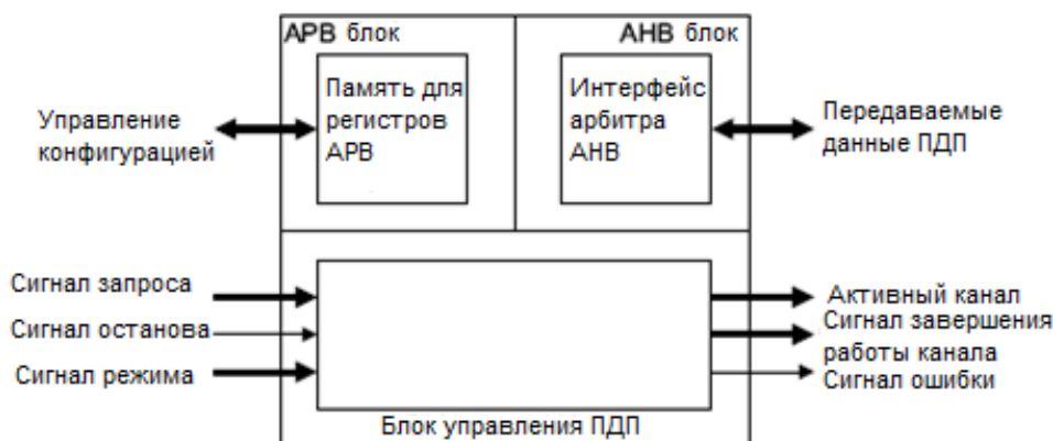
Рисунок 123 – Структурная схема контроллера
