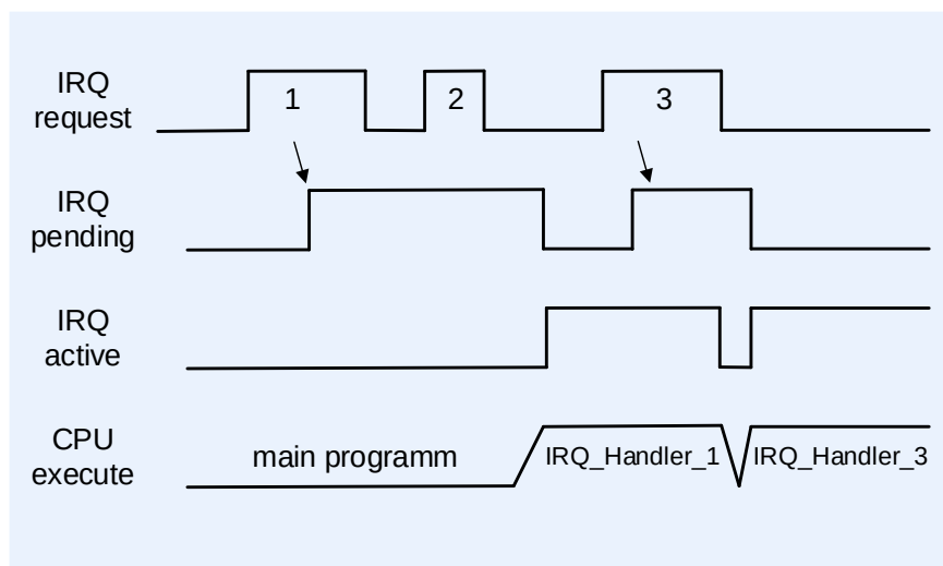
Рисунок 145 – Повторная установка запроса на прерывание в момент выполнения обработчика исключения
