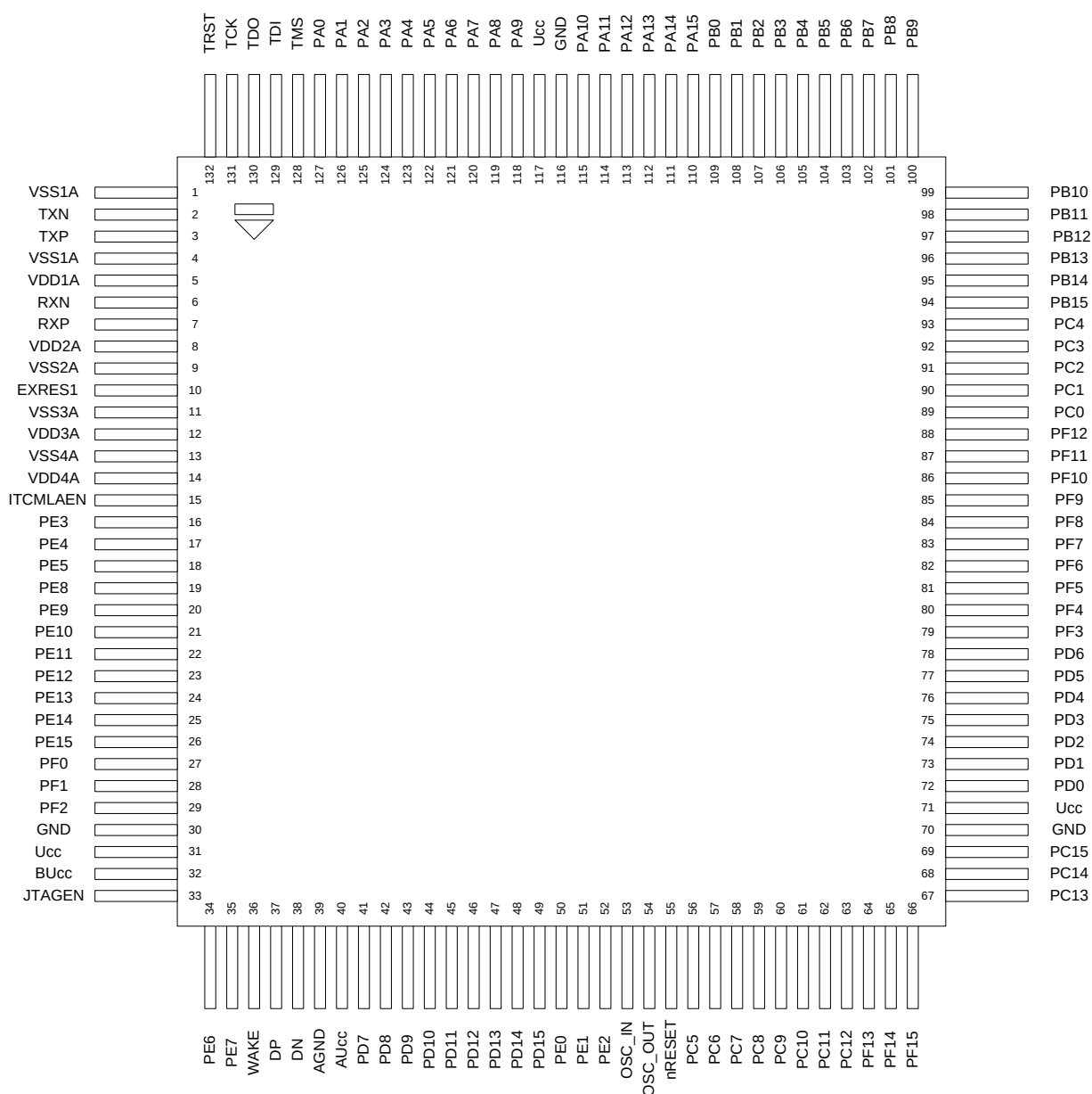
Рисунок 3 – Диаграмма расположения выводов
