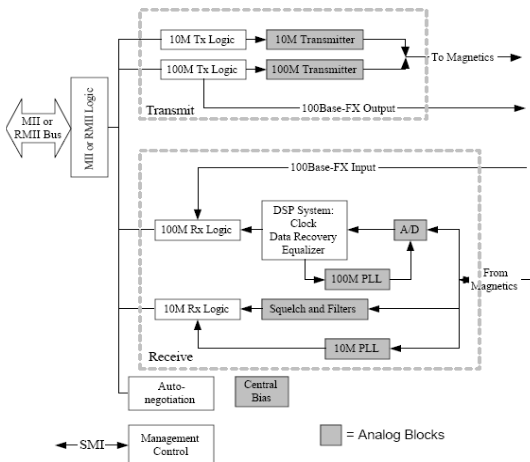
Рисунок 136 – Структурная схема модуля РНУ
