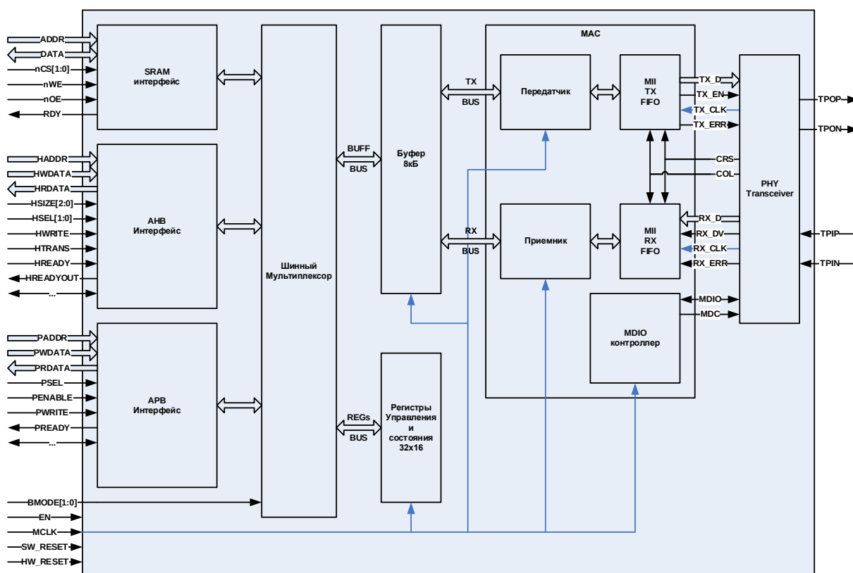
Рисунок 135 – Структурная схема контроллера интерфейса Ethernet
