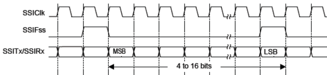
Рисунок 102 – Формат синхронного обмена протокола SSI (непрерывный обмен)
