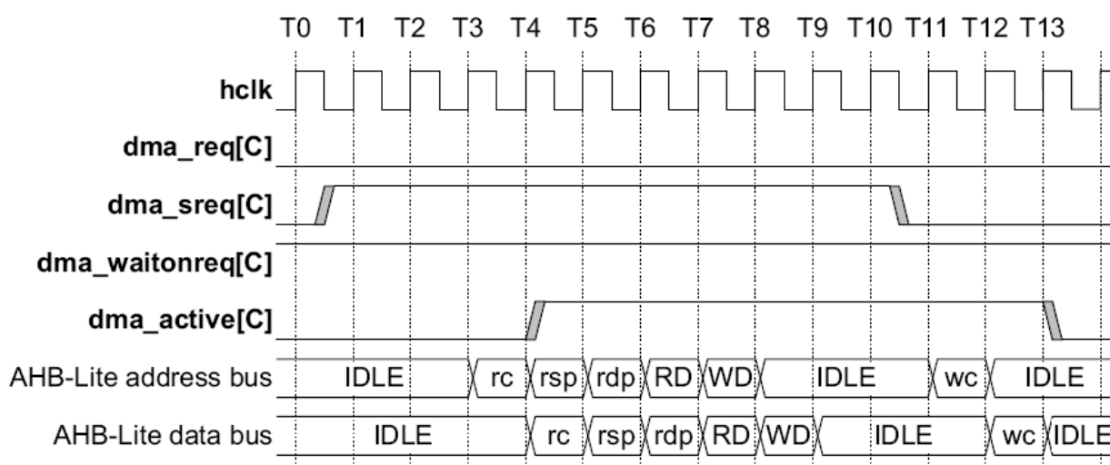
Рисунок 128 – Работа DMA при использовании dma_waitonreq совместно с dma_sreq
