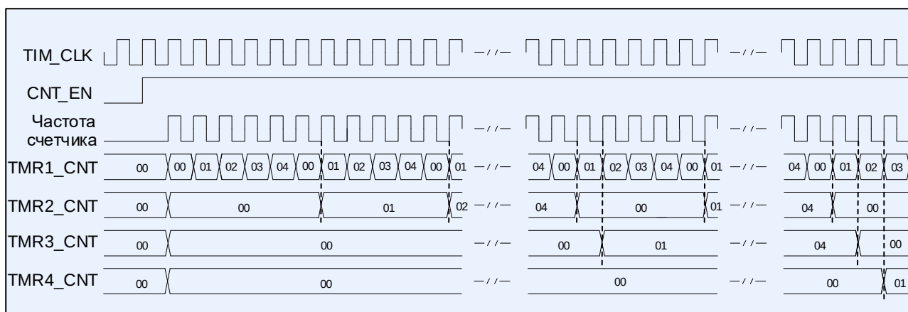
Рисунок 74 – Диаграммы работы четырех таймеров в каскаде
