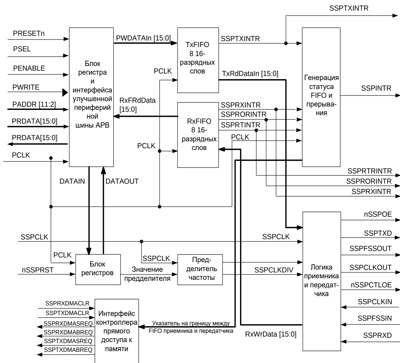
Рисунок 100 – Структурная схема модуля SSP
