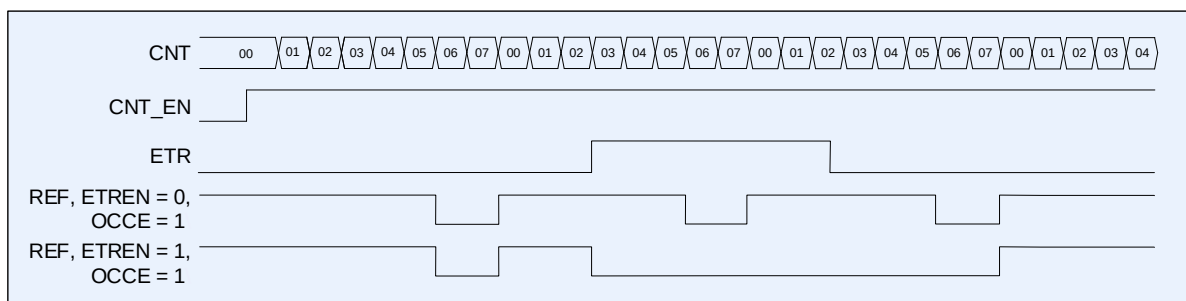
Рисунок 84 – Диаграмма сброса сигнала REF по выводу ETR
