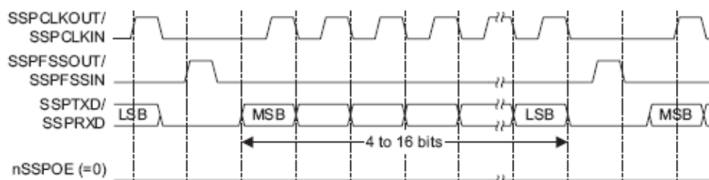
Рисунок 104 – Формат синхронного обмена протокола SPI, SPO=0, SPH=0 (непрерывный обмен)
