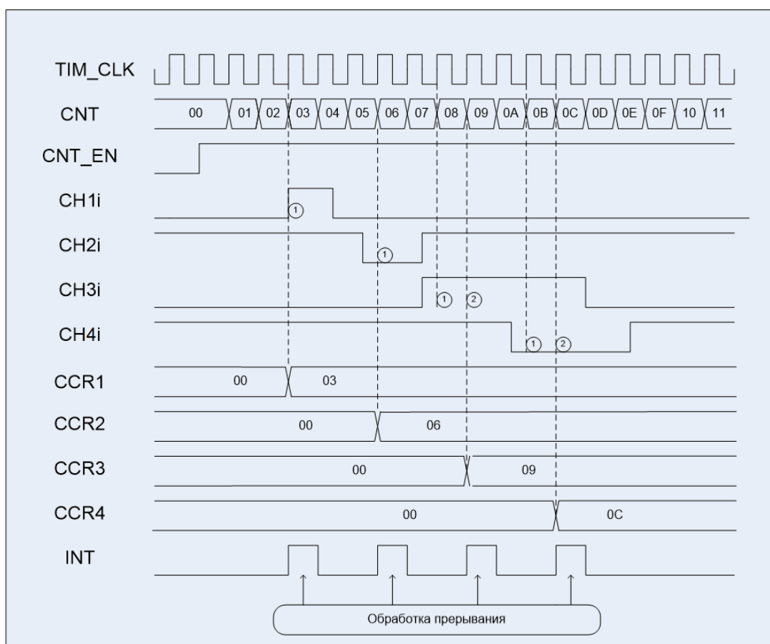
Рисунок 90 – Диаграммы примера работы в режиме захвата
