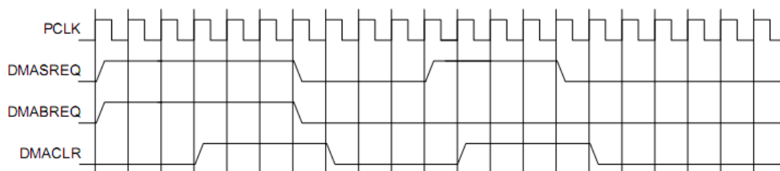
Рисунок 122 – Временные диаграммы одноэлементного и блочного запросов DMA
