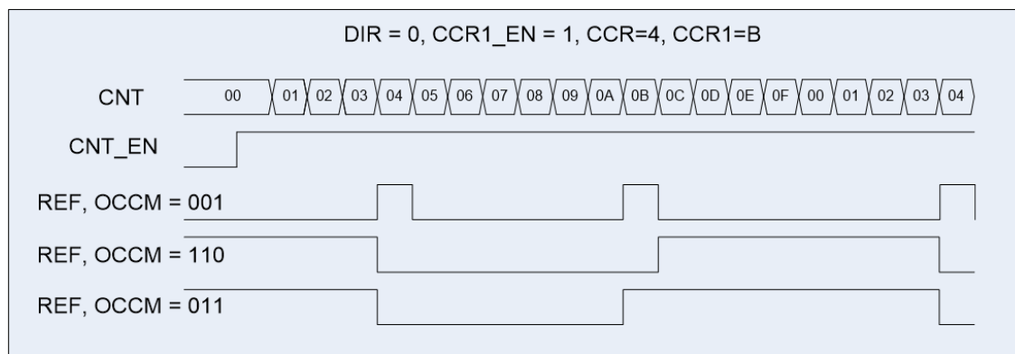
Рисунок 83 – Диаграмма работы в режиме ШИМ, CCR1_EN = 1
