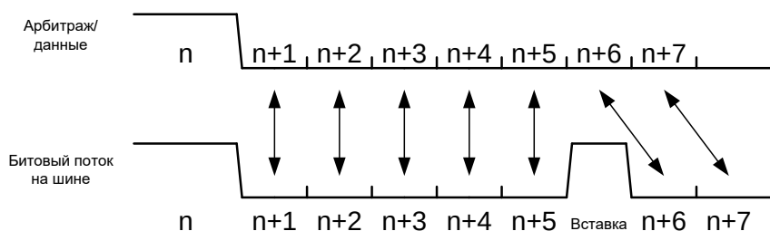
Рисунок 53 – Битстаффинг
