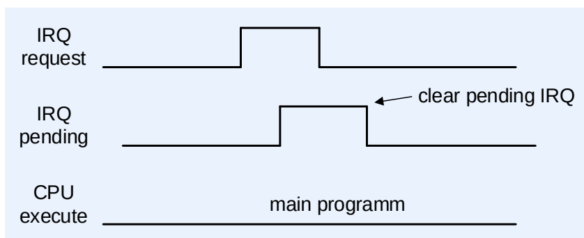
Рисунок 141 – Сброс признака отложенного прерывания, до обработки ядром
