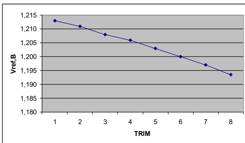
Рисунок 93 – Зависимость источника опорного напряжения от подстройки
