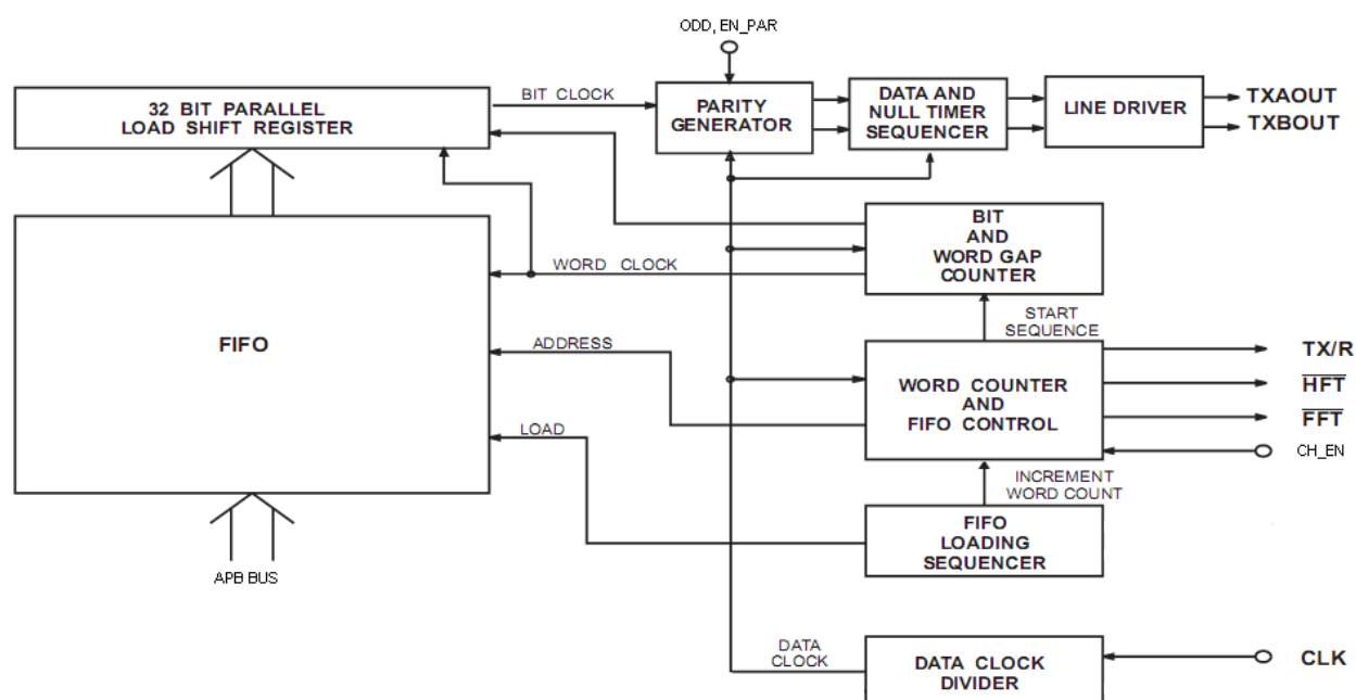
Рисунок 99 – Структурная схема канала передачи
