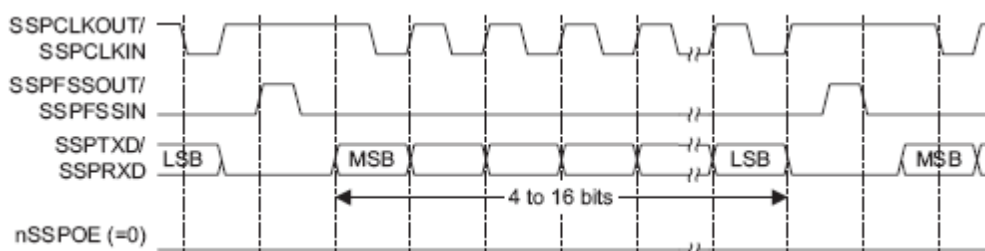
Рисунок 107 – Формат синхронного обмена протокола SPI, SPO=1, SPH=0 (непрерывный обмен)
