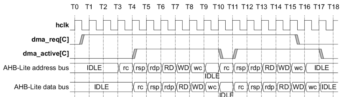
Рисунок 125 – Диаграмма работы при получении запроса на обработку по уровню
