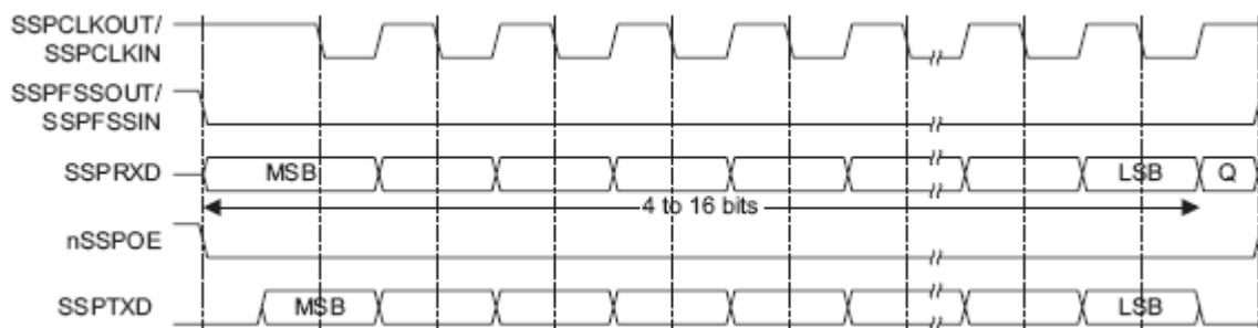
Рисунок 106 – Формат синхронного обмена протокола SPI, SPO=1, SPH=0 (одиночный обмен)
