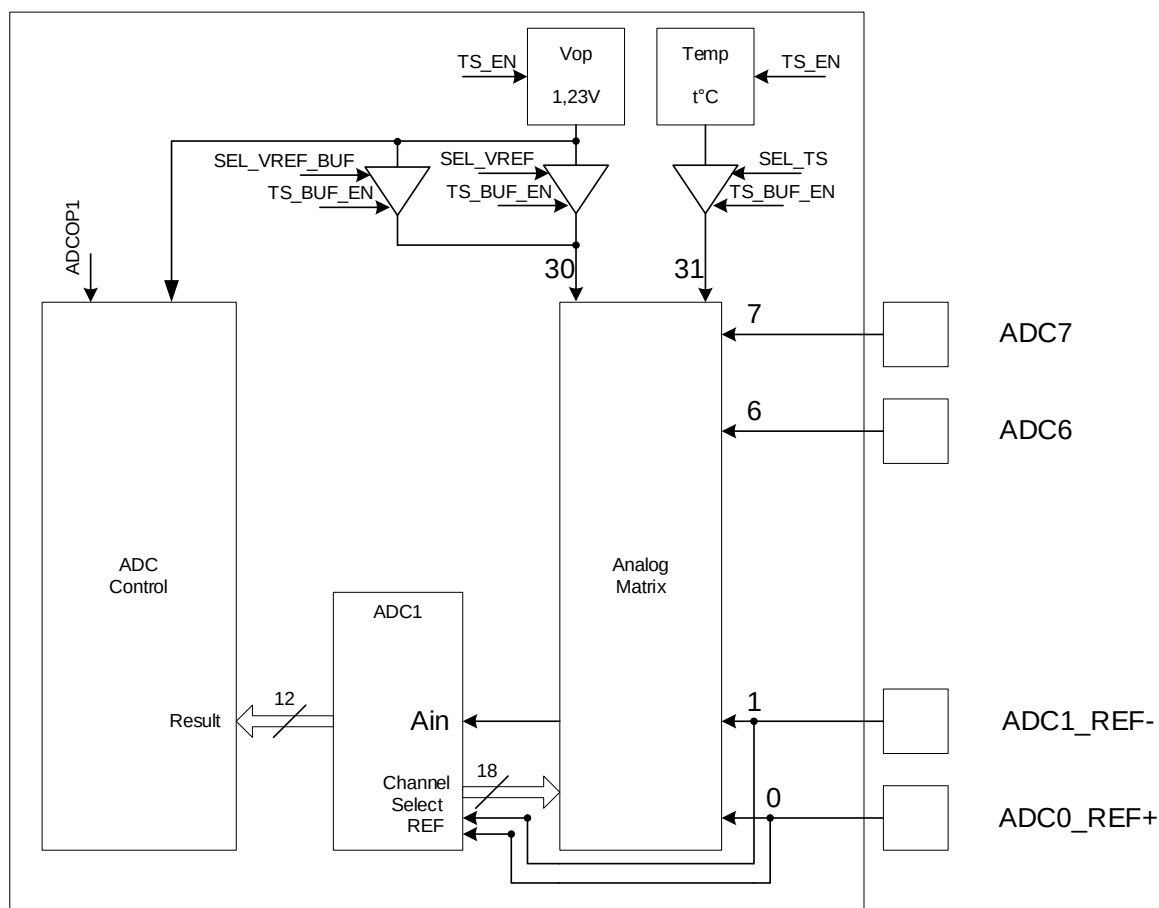
Рисунок 94 – Структурная схема контроллера АЦП
