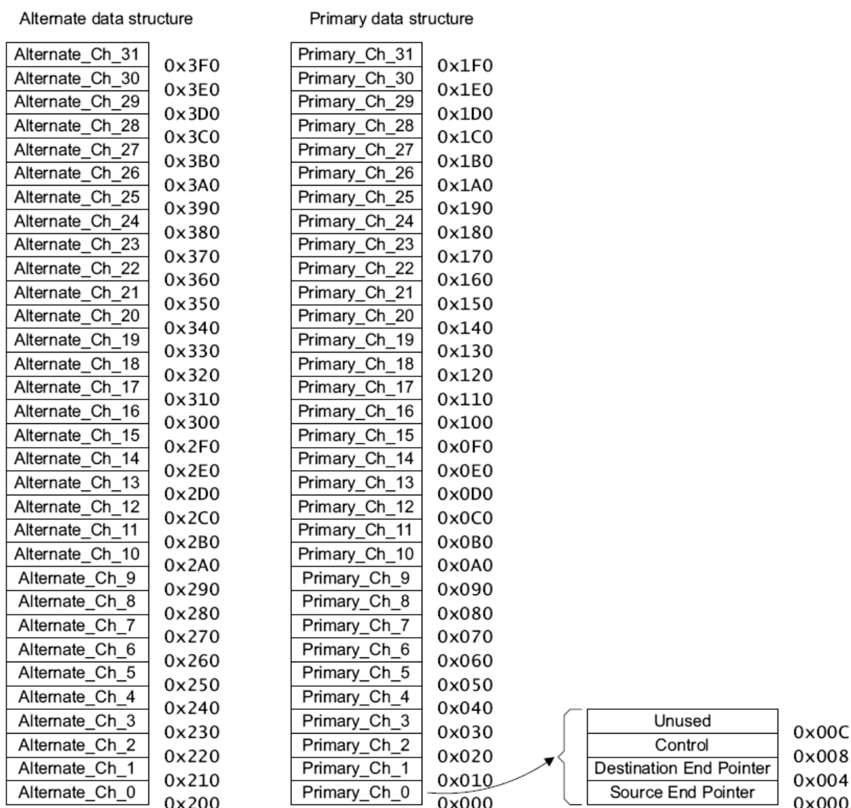
Рисунок 133 – Карта памяти для 32 каналов, включая альтернативную структуру управляющих данных
