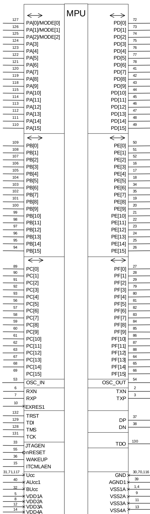
Рисунок 2 – Условное графическое обозначение микросхем
