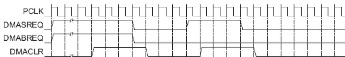
Рисунок 115 – Временные диаграммы обмена в режиме DMA
