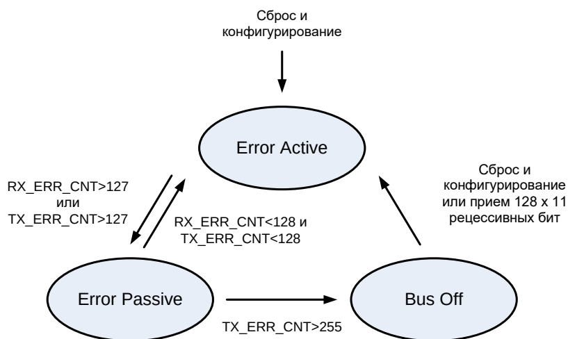
Рисунок 54 – Счетчики ошибок
