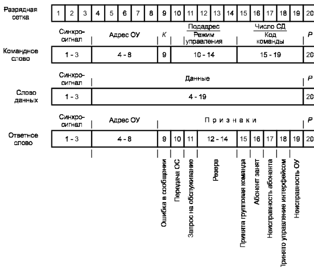
Рисунок 59 – Форматы слов
