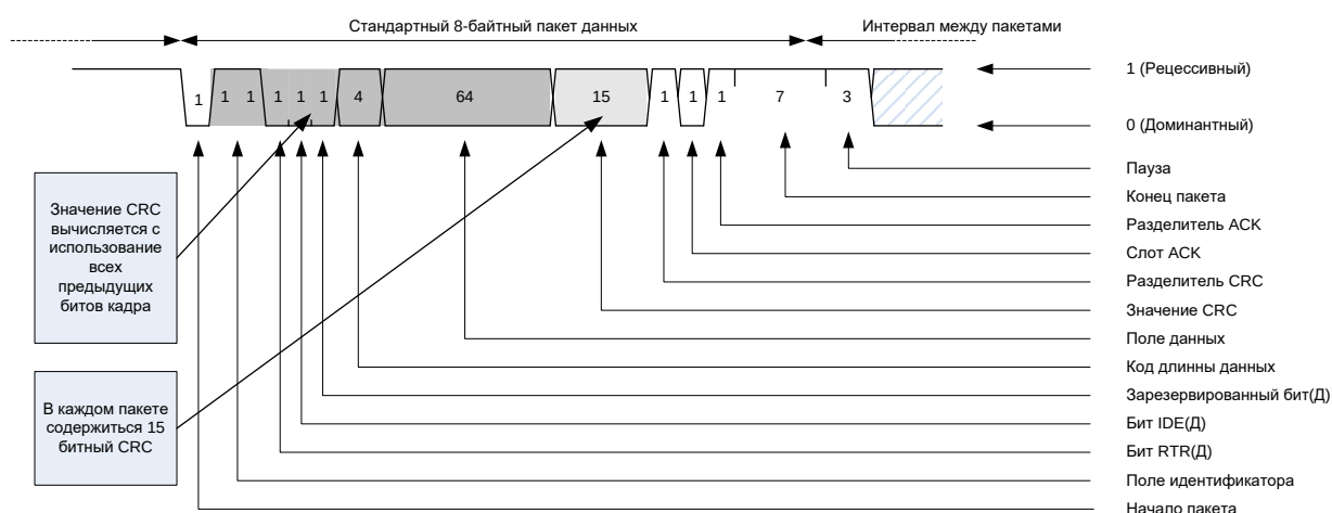
Рисунок 51 – Контроль CRC
