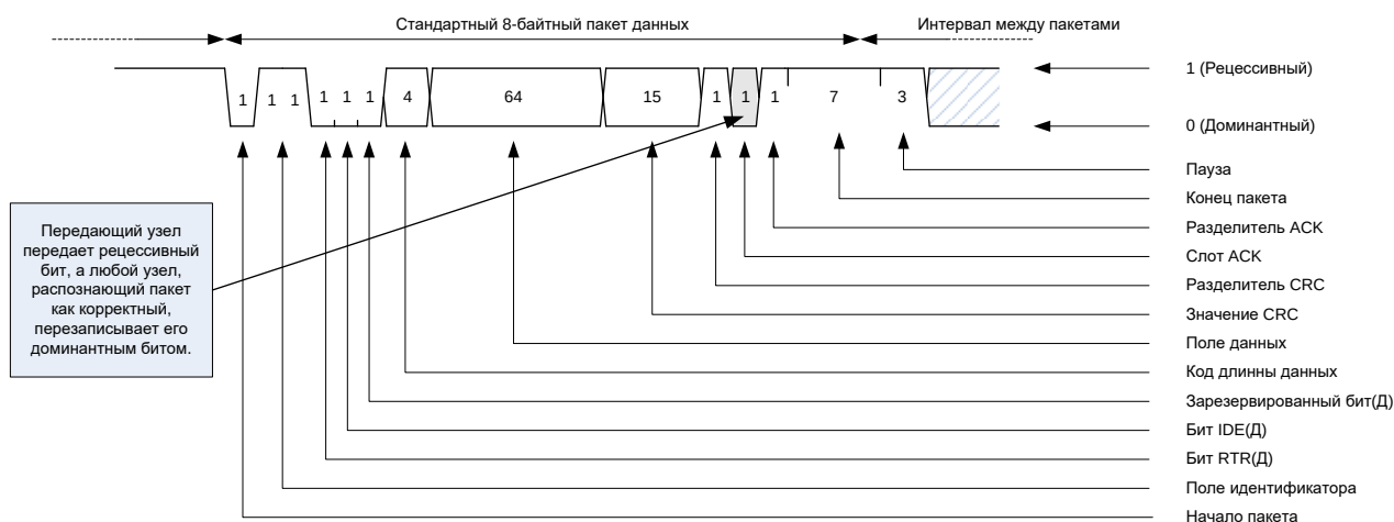
Рисунок 50 – Контроль подтверждения
