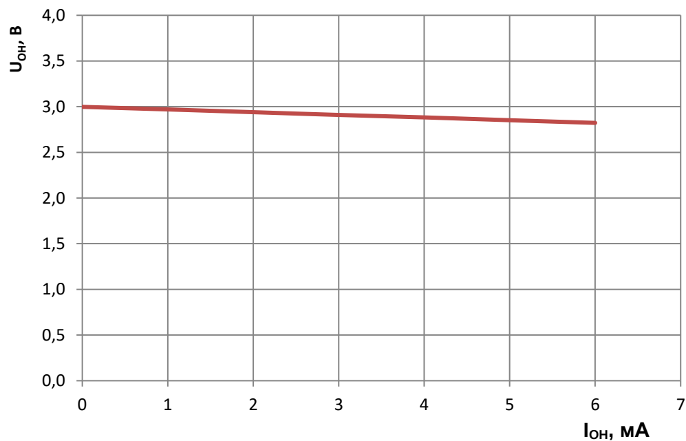
Рисунок 150 – Зависимость выходного напряжения высокого уровня от выходного тока высокого уровня при напряжении питания 3,0 В
