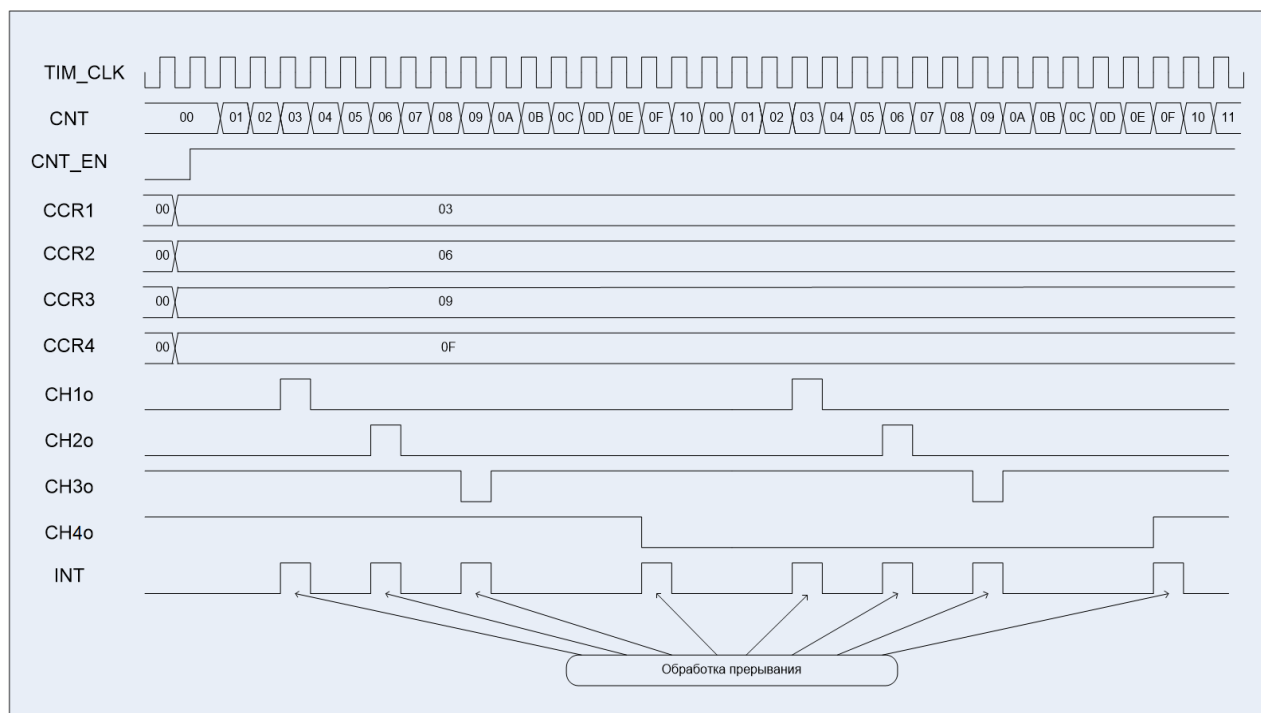
Рисунок 91 – Диаграммы примера работы в режиме ШИМ
